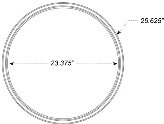
RB-R-24x24 (Riser)
